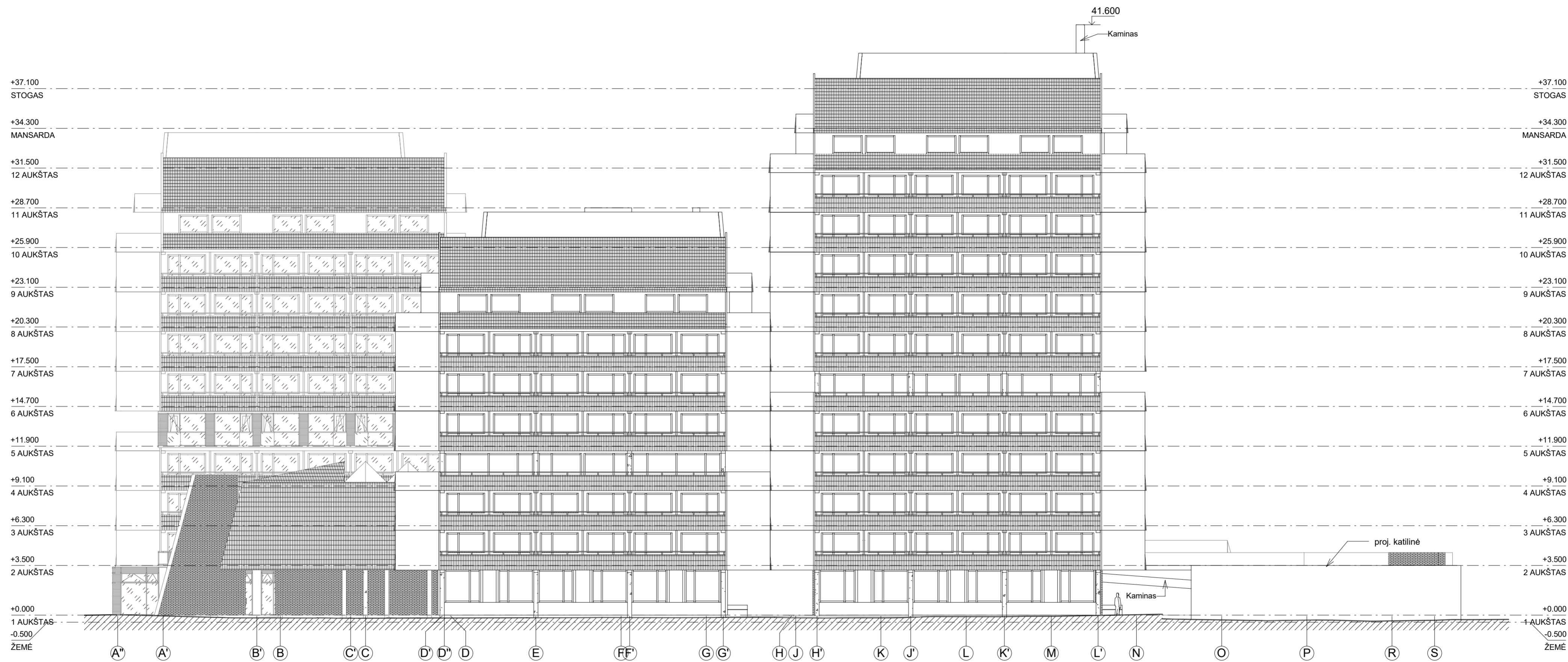
Rytų fasadas ašyje 22, 27 1 : 200
